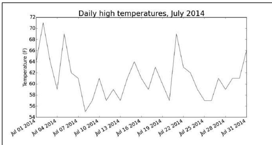
图16-2 现在图表的x轴上有日期，含义更丰富
