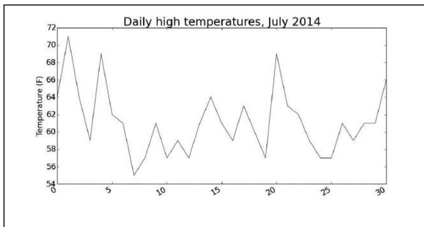
图16-1 阿拉斯加锡特卡2014年7月每日最高气温折线图
