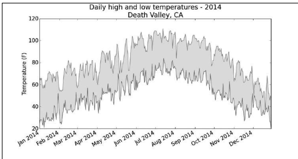
图16-6 死亡谷每日气温和最低气温
